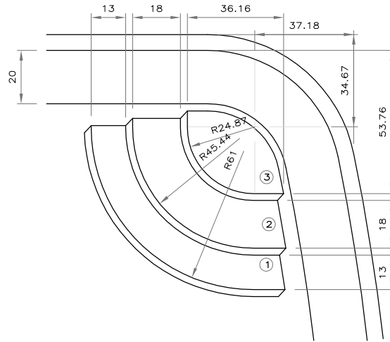
Detalhe Escada Escala 1/20
