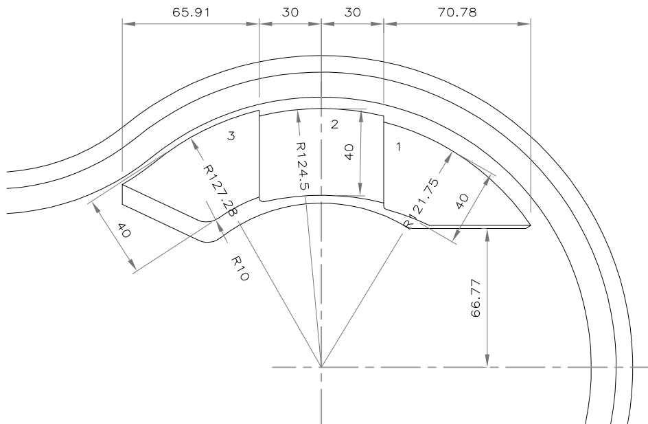
Detalhe degraus Escala 1/25
