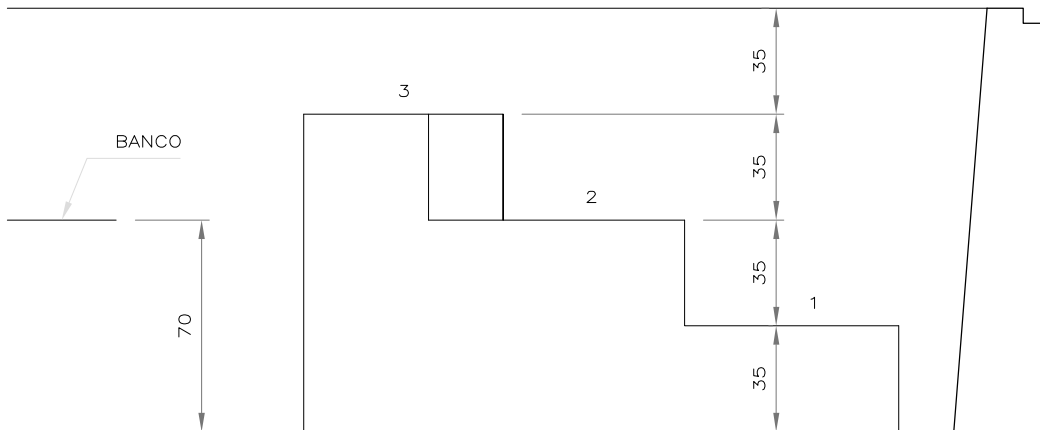
Detalhe degraus Escala 1/25
