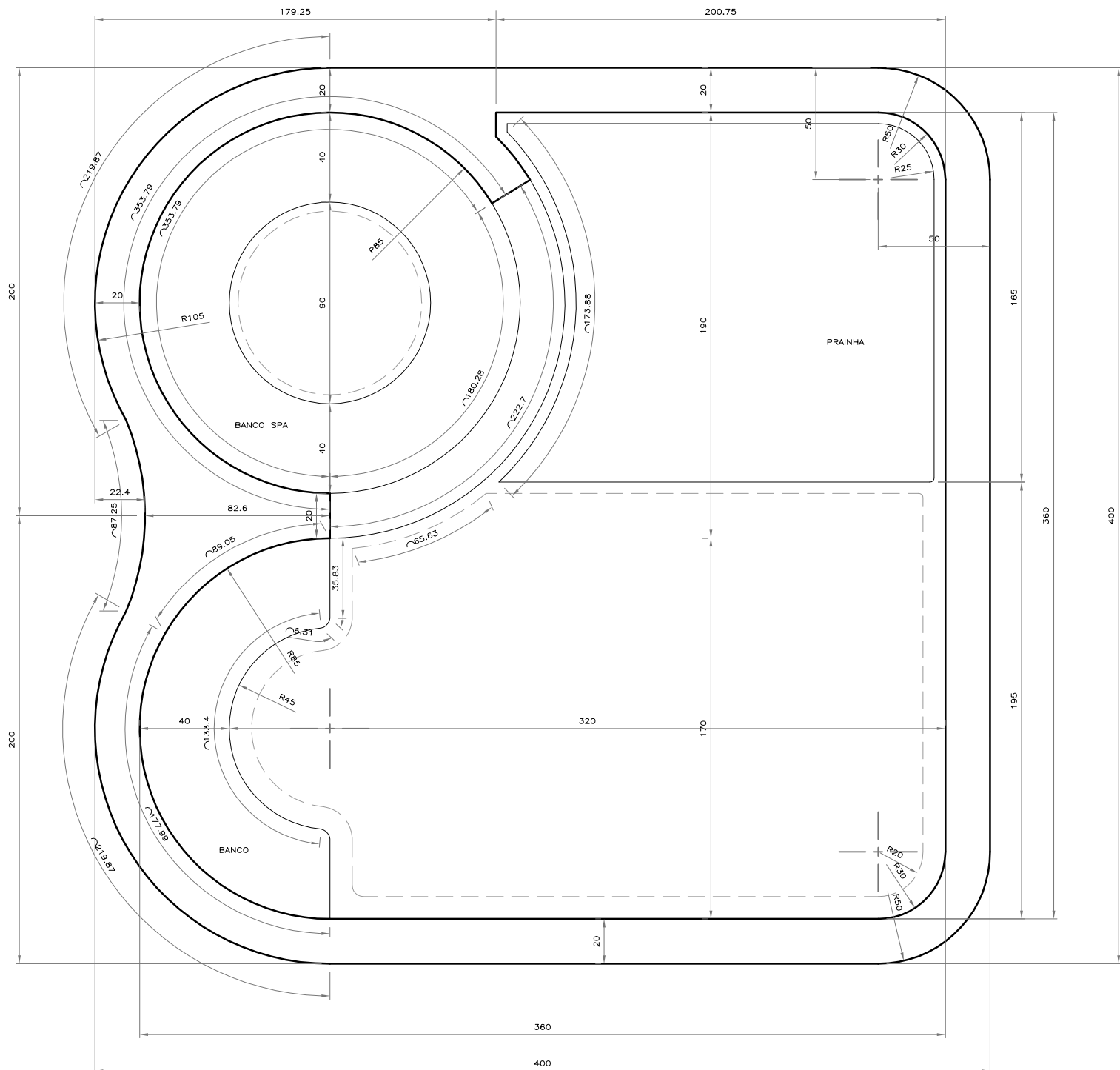
Detalhe degraus e bancos Escala 1/25
