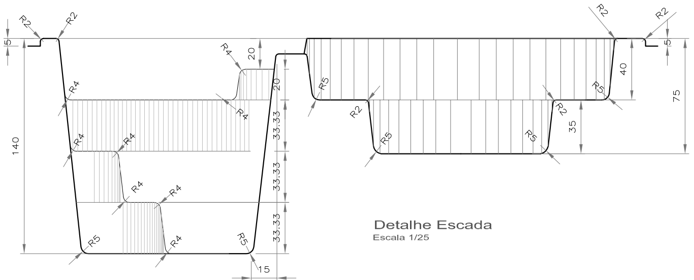
Detalhe Escada Escala 1/25
